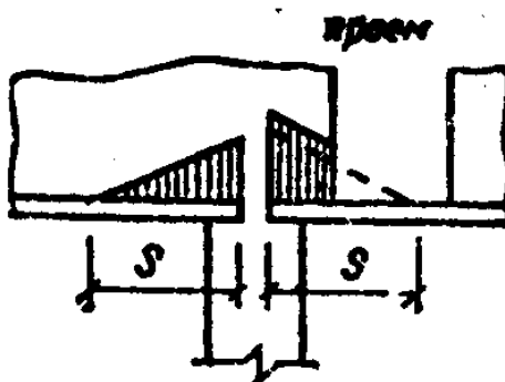
Рис. 16. Эпюра распределения давления в кладке висячих стен при наличии проема
