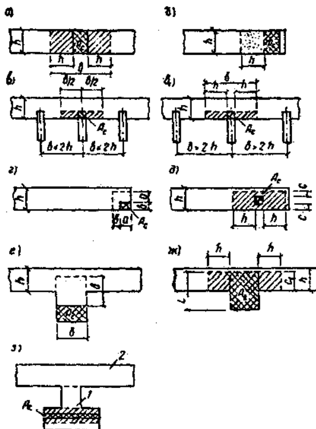
Рис. 9. Определение расчетных площадей сечений при местном сжатии а — з — различные случаи местного сжатия
