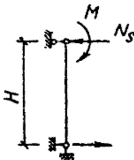
Рис. 12. Определение усилия в анкере от изгибающего момента в уровне перекрытия
