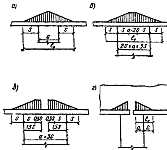
Рис. 15. Распределение давления в кладке над опорами висячих стен
