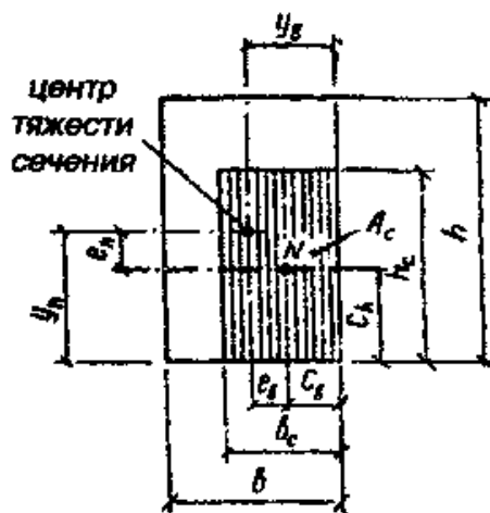
Рис. 7. Расчетная схема прямоугольного сечения при косом внецентренном сжатии
