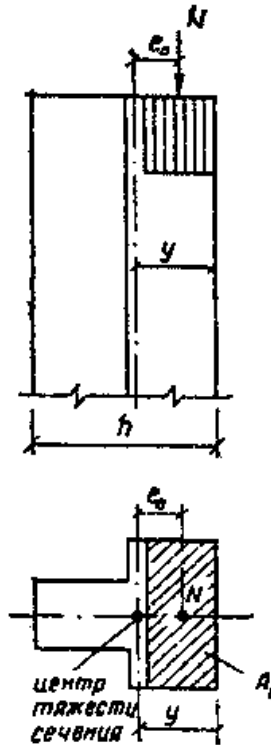
Рис. 5. Внецентренное сжатие
