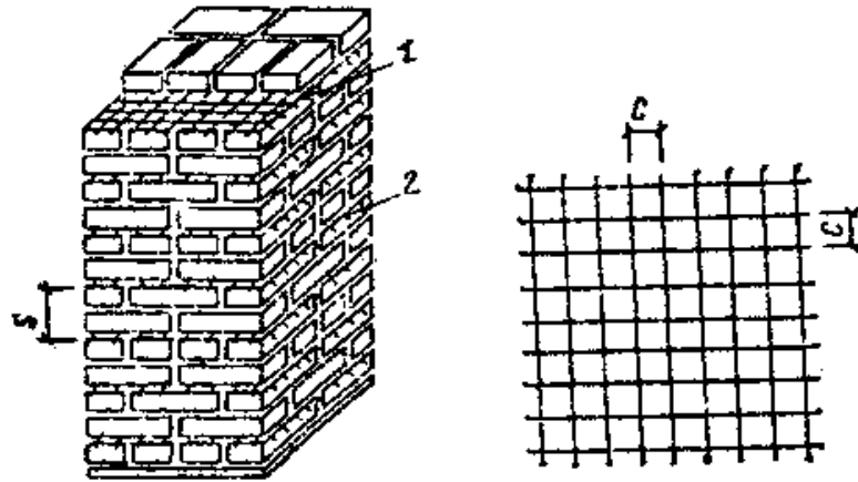
Рис. 10. Поперечное (сетчатое) армирование каменных конструкций 1 - арматурная сетка; 2 - выпуск арматурной сетки для контроля ее укладки
