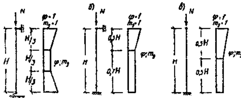
Рис. 4. Коэффициенты \varphi и m_g по высоте сжатых стен и столбов
