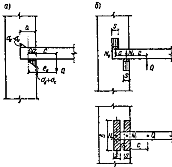
Рис. 14. Расчетные схемы заделки консольных балок
